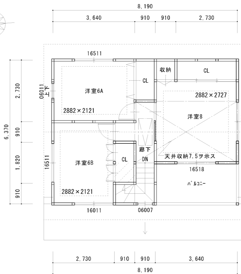
2階 平面図 45.55㎡
