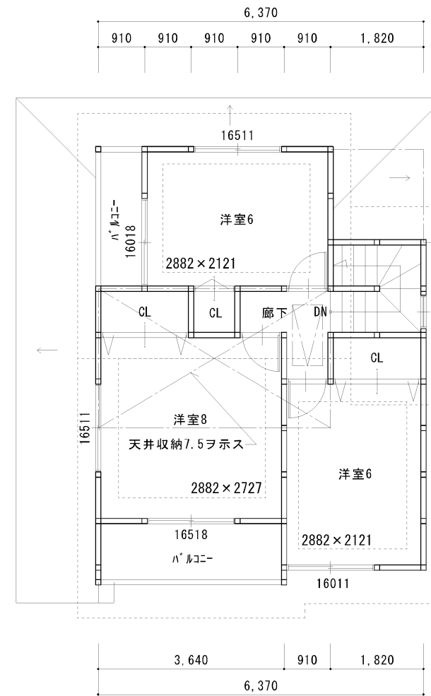
2階平面図
