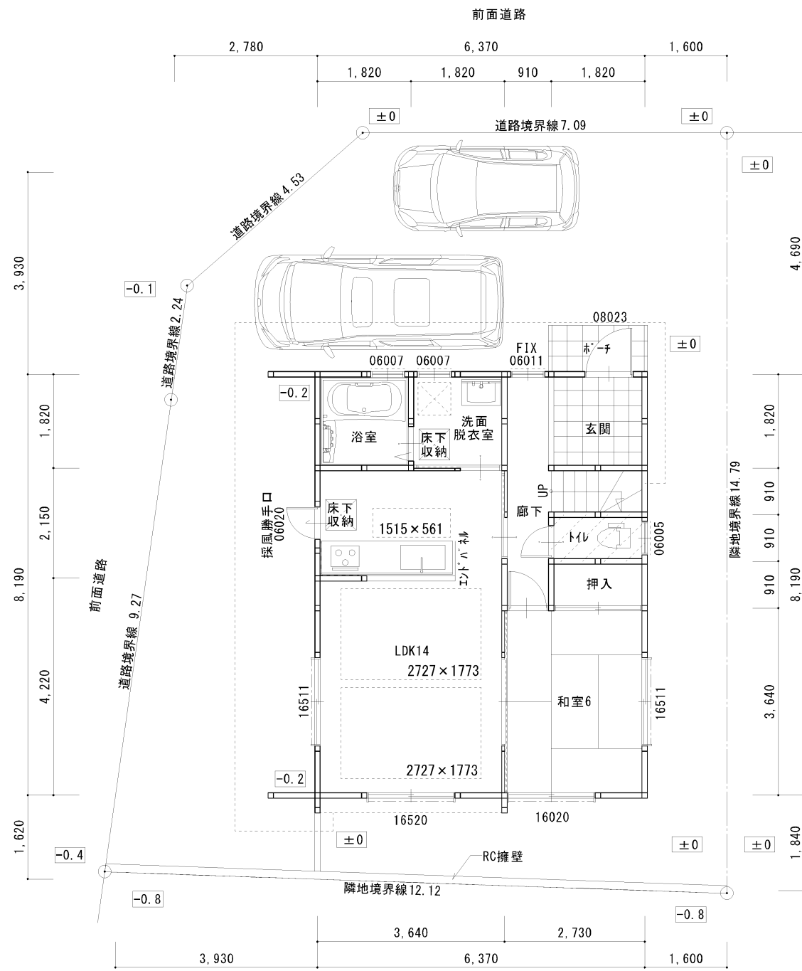
1階平面図
